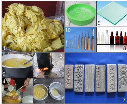
อุปกรณ์ทำเทียนพรรษาประเภทติดพิมพ์
